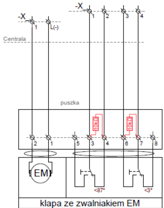
Rys. 21. Schemat siłownika ze zwalniającym elektromagnetycznym.
