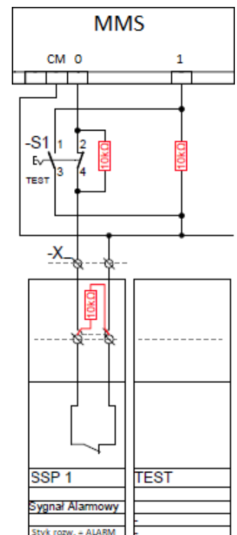
Rys. 23. Schemat podłączenia sygnału SSP.
